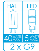
CG0504B-2WH WHITE FINISH ACABADO EN BLANCO SIZE / TAMAÑO (CM) W36.5 X E7.4 X H11
